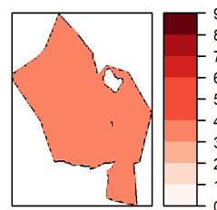
DyDs ANN RCP 8.5 (3.6 °F)
