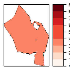
DyDs ANN RCP 4.5 (3.5 °F)
